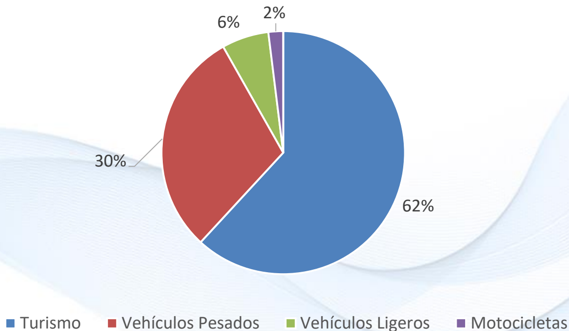
Emisiones por categoría de vehículos (% total de emisiones de CO 2 -eq de transporte carretera)
